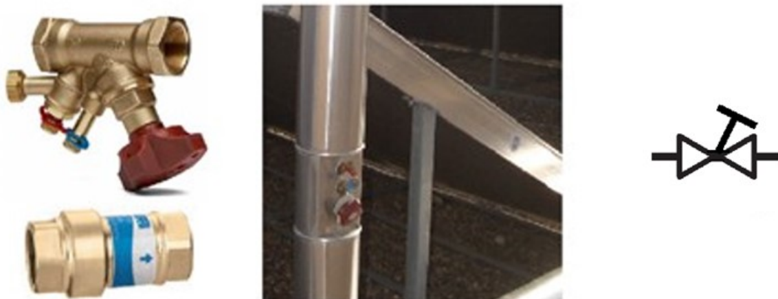
Figura 78: Dos tipos de válvulas de equilibrado, instalada con mando accesible y símbolo habitualmente utilizado
