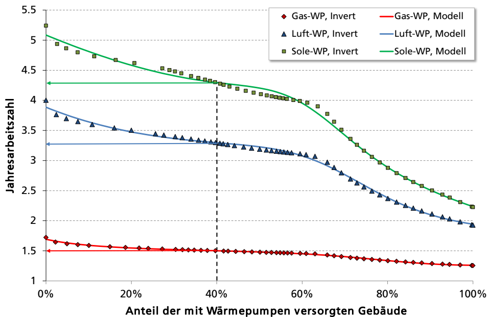
Abb. 7 Mittlere Jahresarbeitszahl von Wärmepumpen in Abhängigkeit des Anteils aller Gebäude, die durch Wärmepumpen mit Wärme versorgt werden. Die Punkte resultieren aus Ergebnissen von Invert-Rechnungen /Invert, 2013-II/ und die Linien stellen die Funktionen dar, mit denen in den REMod-D-Rechnungen gearbeitet wurde. Zu den Beispielwerten siehe im Text.
